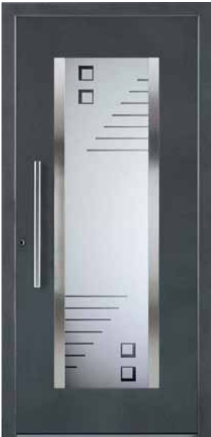
LA 540 flügelüberdeckend Edelstahapplikation flächenbündig Farbe: ST 703 dunkelgrau Glastype: 540.7242 Klarglas teilmattiert Linien klar Griff: 0101 E (600 mm)
