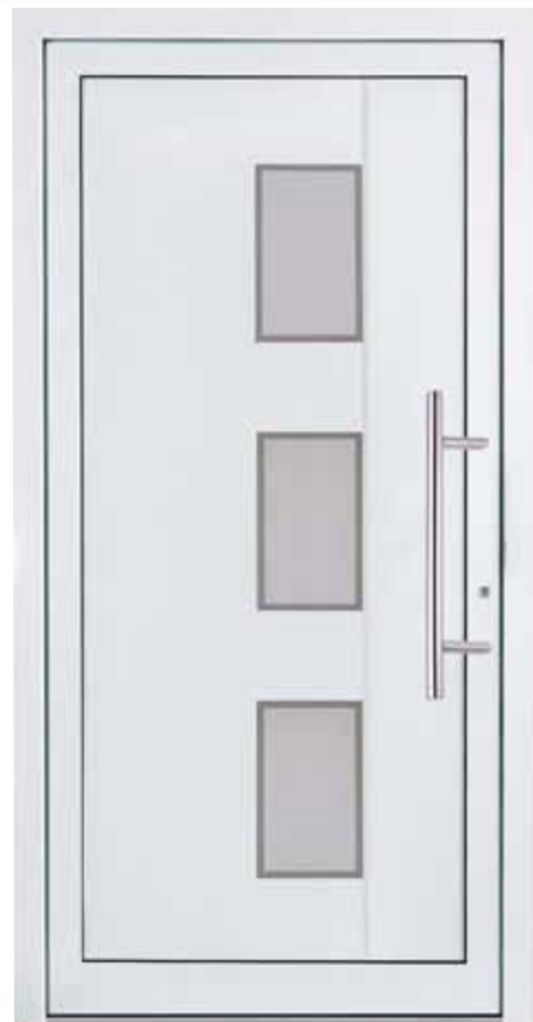
LAN 940 mit Nutenfräsung außen Farbe: weiß · Glasstyp: 940.7001 S Klarglas teilmattiert Rand umlaufend klar · Griff: 0103 E-600 S
