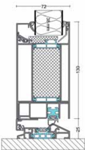
Dämmwertberechnung: Profil W72 mit Mitteldichtung Türfüllung mit 2-fach Verglasung U_D ca.: 1,1 W/m 2 K
